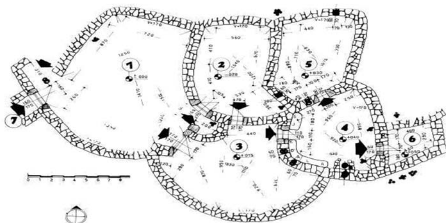
Tlocrt Dudićevog osika (Konzervatorski odjel u Rijeci, 1975.)
